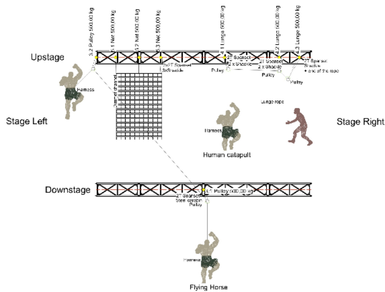
2 Rigging front Scale: 1:100
